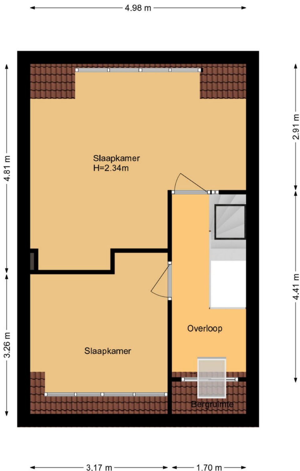
2e Verdieping
